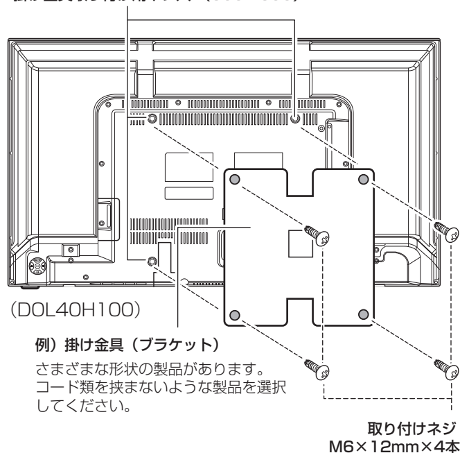
掛け金具取り付け用ネジ穴（300×300）
