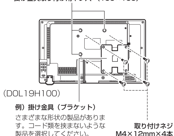
掛け金具取り付け用ネジ穴（100×100）
