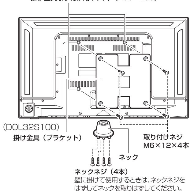
掛け金具取り付け用ネジ穴（200×200）
