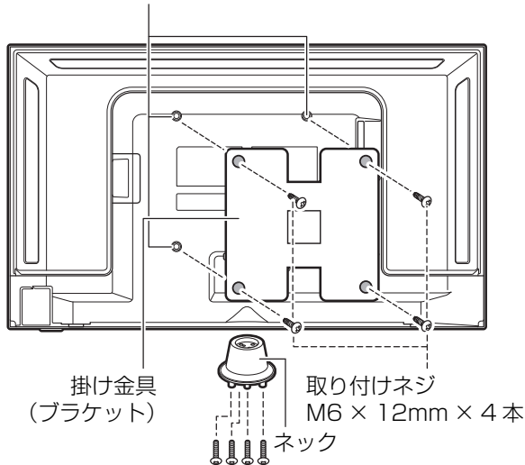
掛け金具取り付け用ネジ穴 (200 × 200)
