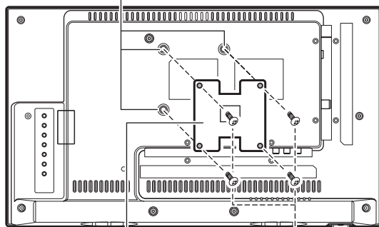
掛け金具取り付け用ネジ穴（75×75）
