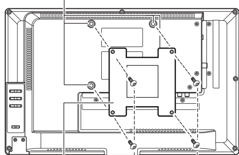
掛け金具取り付け用ネジ穴（100×100）
