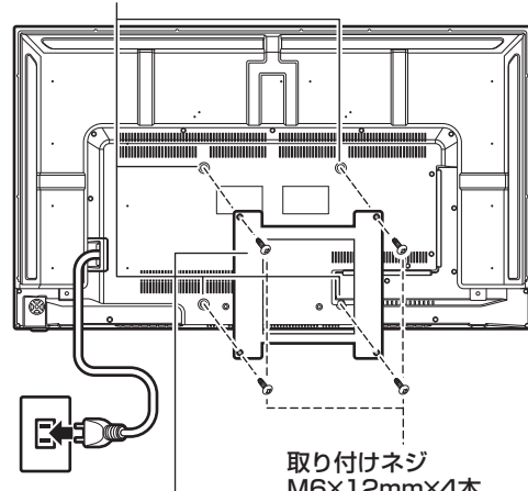
掛け金具取り付け用ネジ穴 (300×300)
