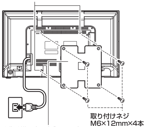
掛け金具取り付け用ネジ穴 (200×300)
