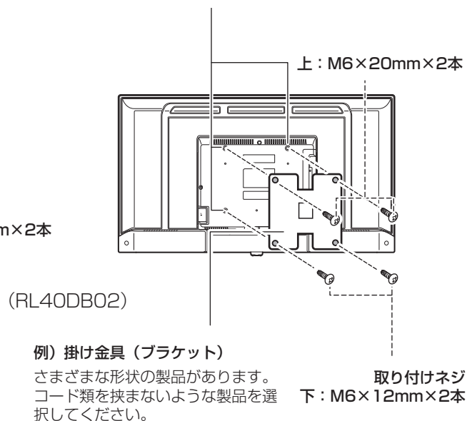
掛け金具取り付け用ネジ穴（200×200）
