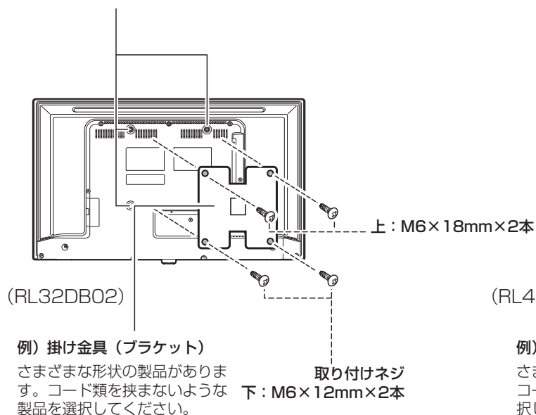
掛け金具取り付け用ネジ穴（200×200）
