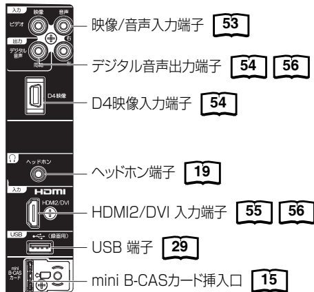
イラスト: RN-24DG10/RN-32DG10/RN-40DG10
