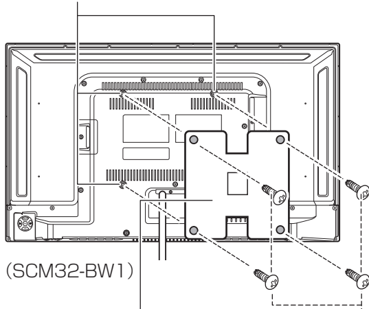
掛け金具取り付け用ネジ穴 (200×200)
