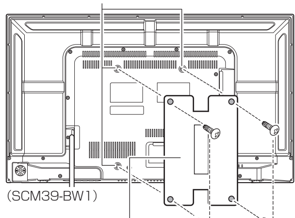
掛け金具取り付け用ネジ穴 (200×300)
