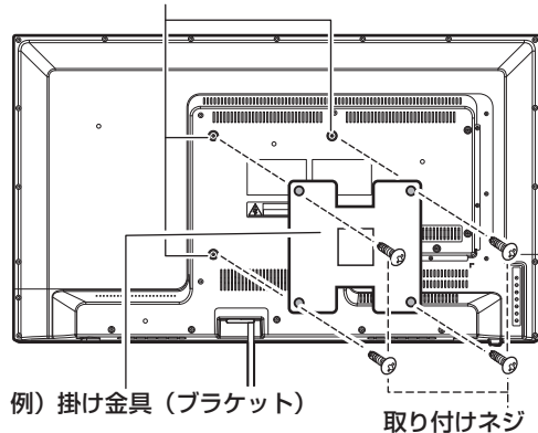
掛け金具取り付け用ネジ穴 (200×200)
